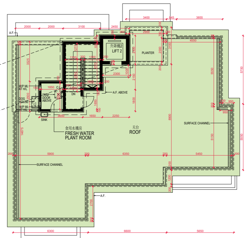
R/F FLOOR PLAN 天台樓面平面圖
